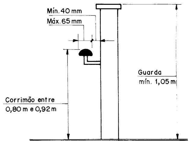
Figura 15 - Dimensões de guardas e corrimãos
