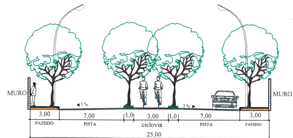
SEÇÃO TIPO
