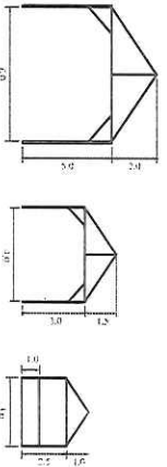
ELEVAÇÃO BARRACAS
